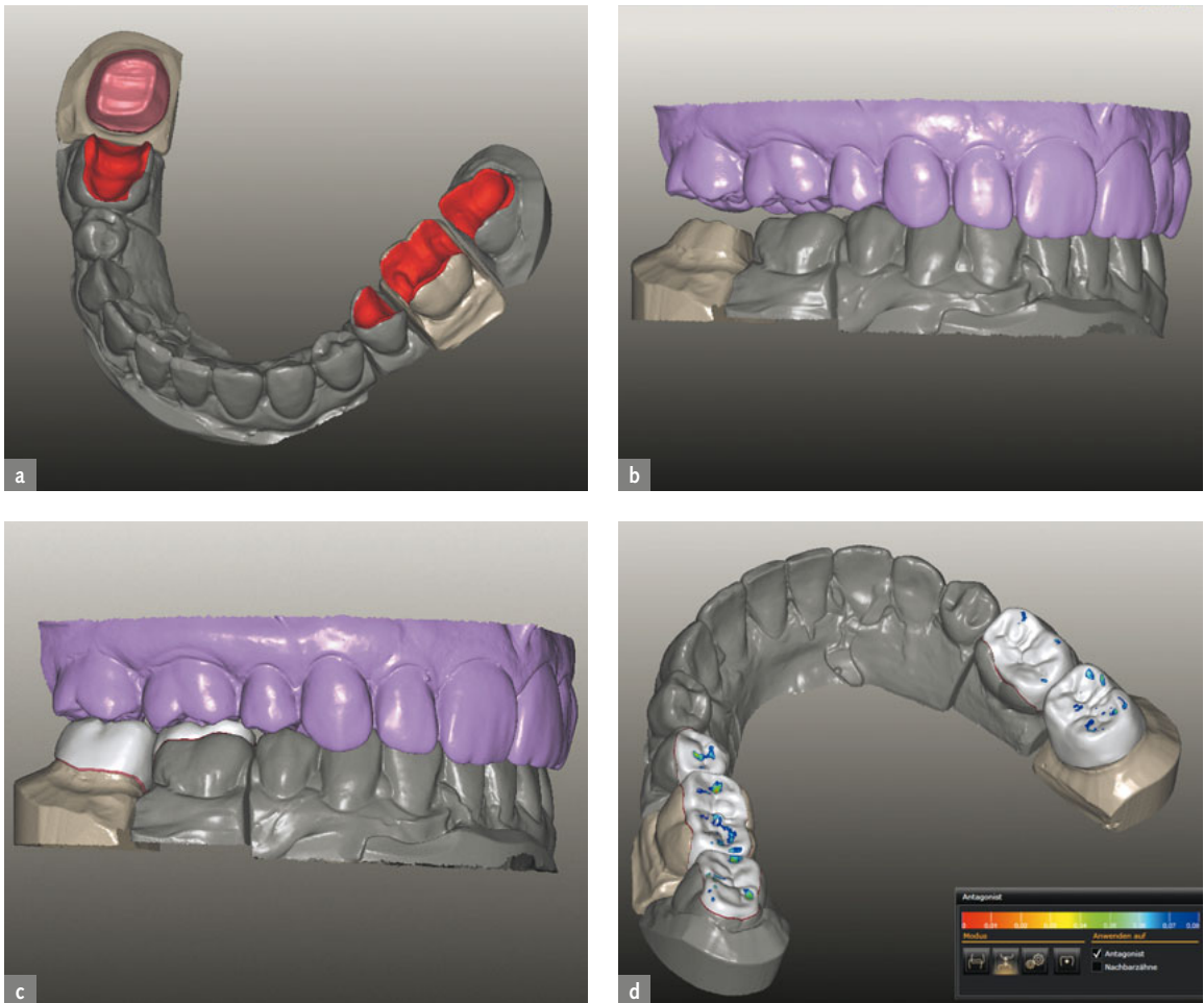
Abb. 31a bis d Schritte der digitalen Planung: eingescanntes Unterkieferpräparationsmodell (a). Die Präparationsgrenzen werden automatisch erfasst. Dimensionsgenaue Orientierung zum Oberkiefer (b). Automatisches Design der Versorgung (c). Optimierung der Kontaktbeziehungen (d).
