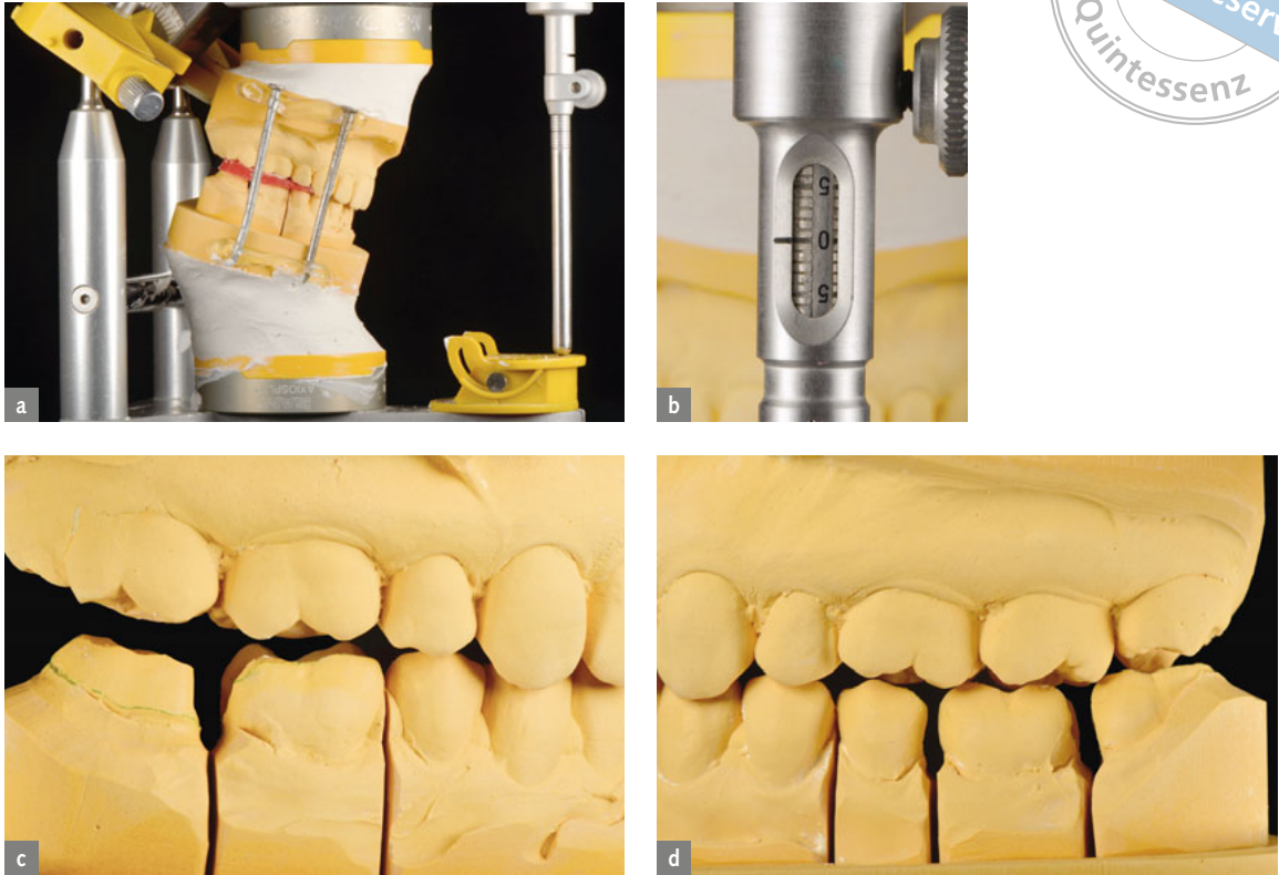
Abb. 30a bis d Die Sägemodelle sind in der therapeutischen Kieferrelation und Vertikaldimension montiert, vorbereitet zum Scannen durch die Zirkonzahn-Technologie.
